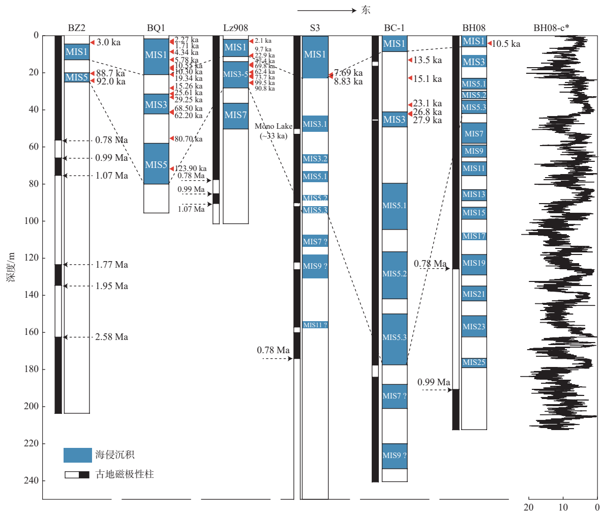
图 4 渤海海域第四纪海侵对比
