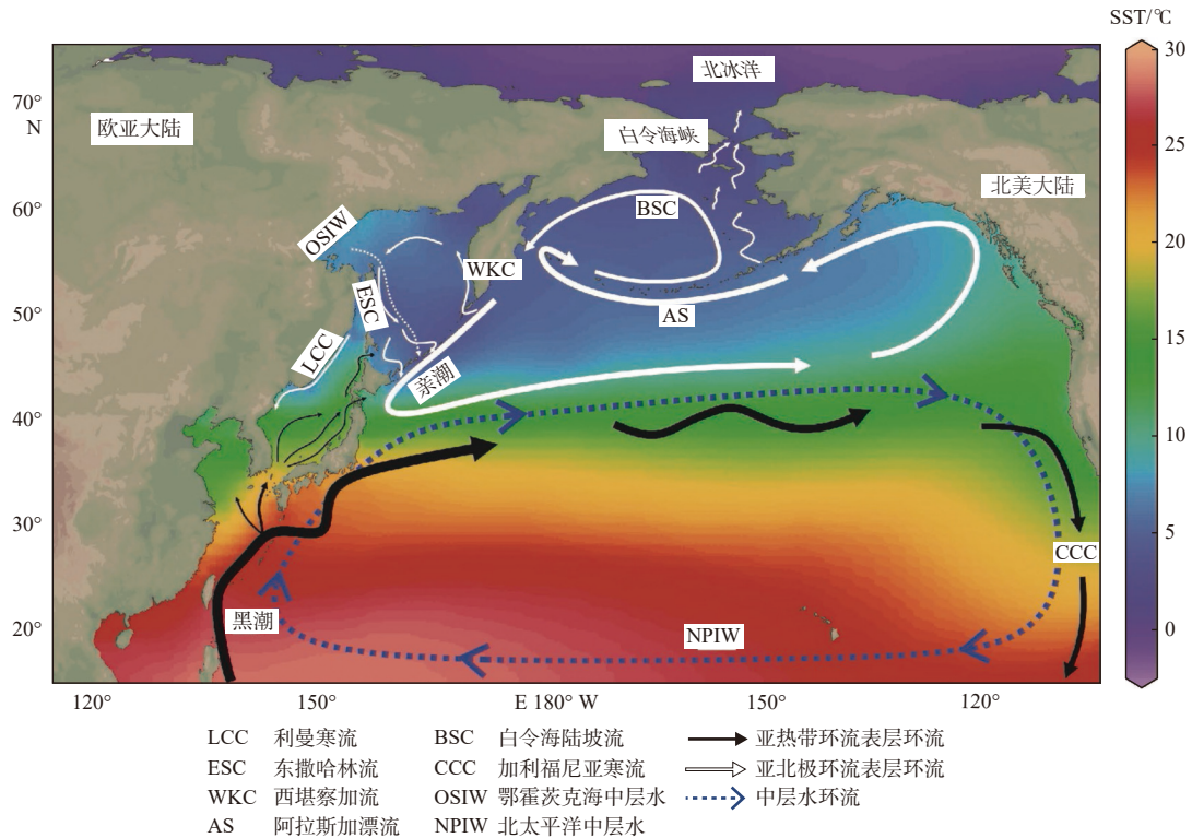
图 3 西北太平洋年均表层海水温度、表层环流和北太平洋中层水
