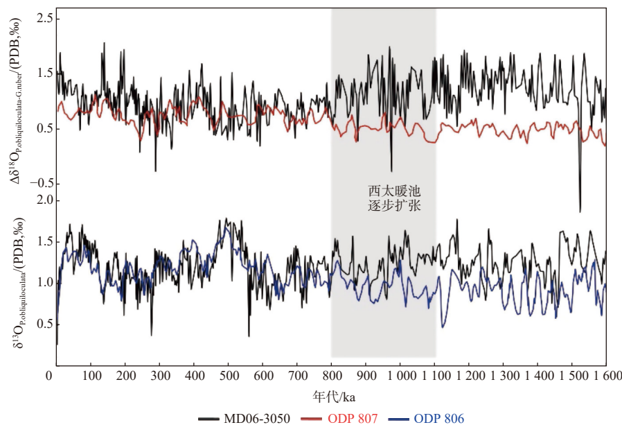
(b) 浮游有孔虫氧碳同位素反映的在1.1—0.8 Ma期间逐渐趋同的暖池的核心和边缘区水文环境
