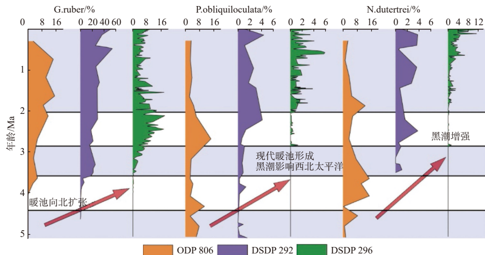
(a) 浮游有孔虫群落组成反映的西太暖池对西北太平洋的影响
