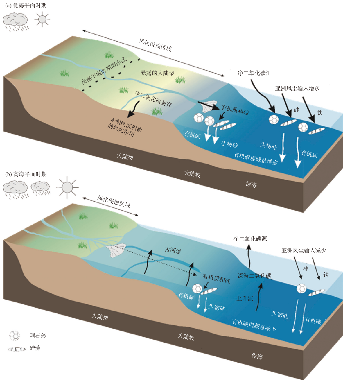
图 5 第四纪冰期旋回中黑潮源区周边的陆表风化剥蚀作用过程及其产物入海的碳循环效应
